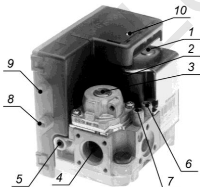
Рисунок 10. Газовый клапан с контроллером
