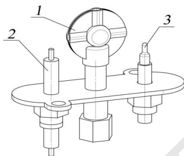
1 – трехпламенная головка; 2 - электрод розжига; 3 – термопара.
