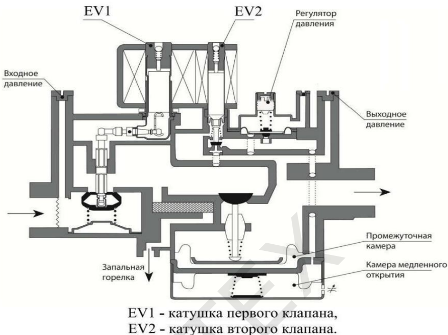
Рисунок – 3. Устройство газовой автоматики
