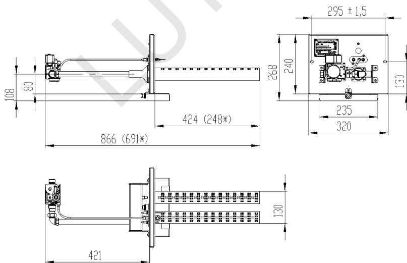
Рисунок – 1. Общий вид газогорелочного устройства.
